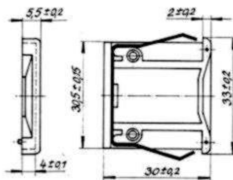
Bočnice vnější WF 251 00 (šedá), WF 251 39 (černá)
